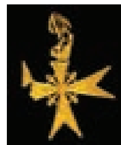
ЧАСТ ОТ СЪКРОВИЩЕТО НА ПОТЪНАЛ ИСПАНСКИ КОРАБ
