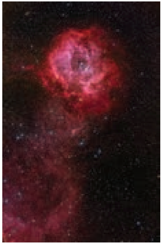
ГОРЕ ЛЯВО: ТРИЪГЪЛНАТА ГАЛАКТИКА (M33) / ГОРЕ ДЯСНО: МЪГЛЯВИНАТА РОЗЕТКА (NGC 2237) ДОЛУ ЛЯВО: МЪГЛЯВИНА NGC 3582 В МЛЕЧНИЯ ПЪТ / ЦЕНТЪР: МЪГЛЯВИНА В СЪЗВЕЗДИЕТО КЕНТАВЪР (RCW 79) ДОЛУ ДЯСНО: МЪГЛЯВИНАТА ЛЕБЕД
